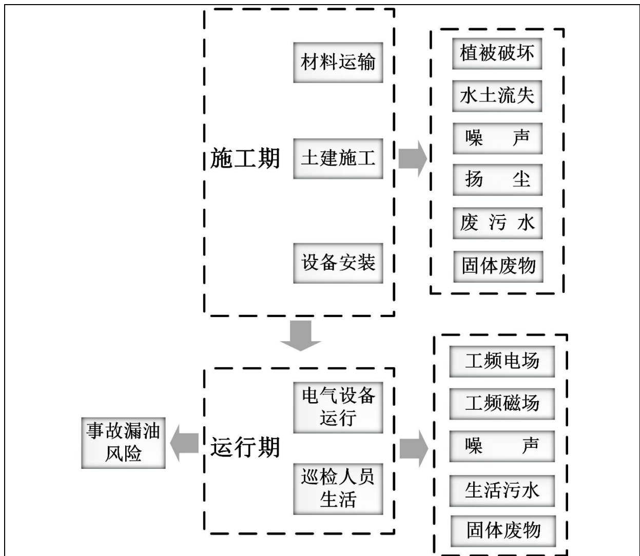
图 8 变电站工程施工期和运行期的产污节点图
