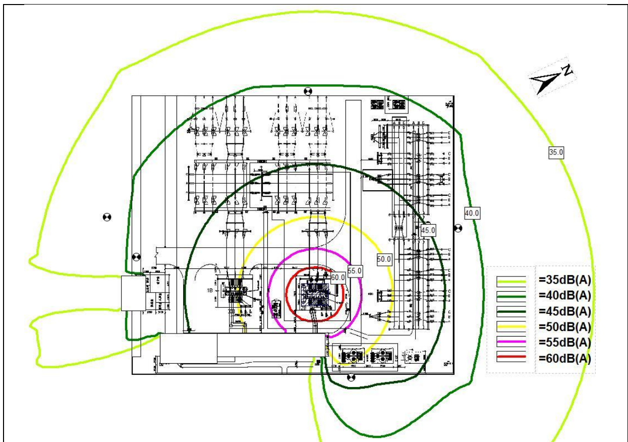
图 9 温塘 110kV 变电站本期规模噪声预测等值线图
