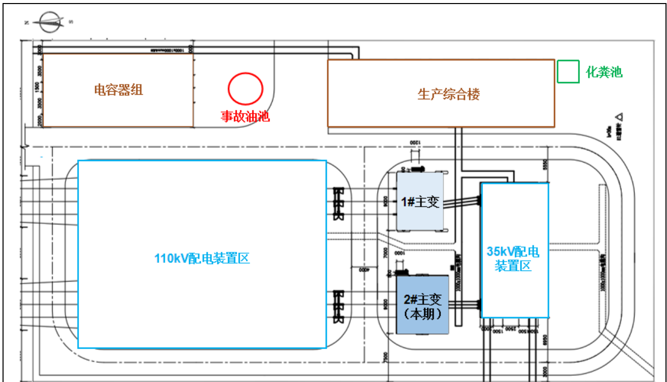
图 1-2 青麓 110kV 变电站总平面布置图
